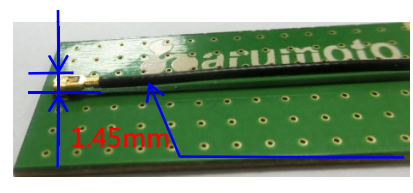
OD 0.95 / 1.13 / 1.32 / 1.37mm
