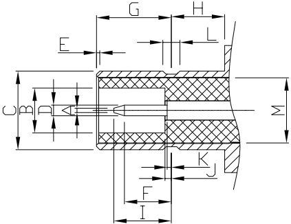
插座 Jack
