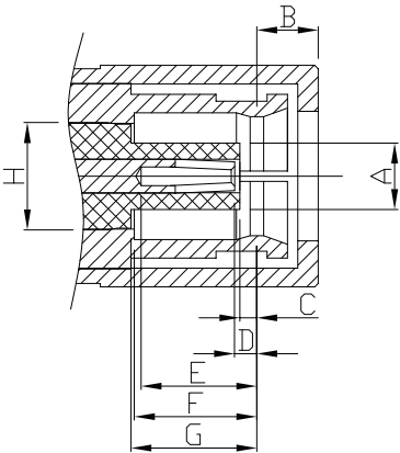
插头 Plug
